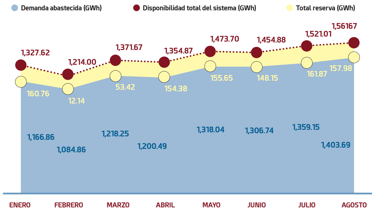
ILUSTRACIÓN 6. DISPONIBILIDAD, DEMANDA ABASTECIDA Y RESERVA DEL SISTEMA ELÉCTRICO NACIONAL INTERCONECTADO (SENI) ENERO-AGOSTO DE 2017
